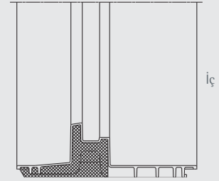
Değişken kasa profil kesiti
